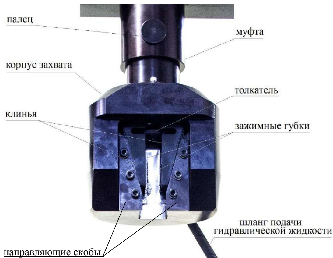
Рисунок 3 – Общий вид клинового захвата
